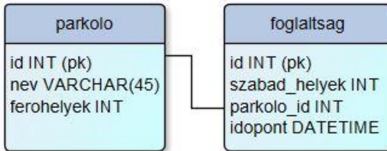
15. Ábra Az adatbázis struktúrája
