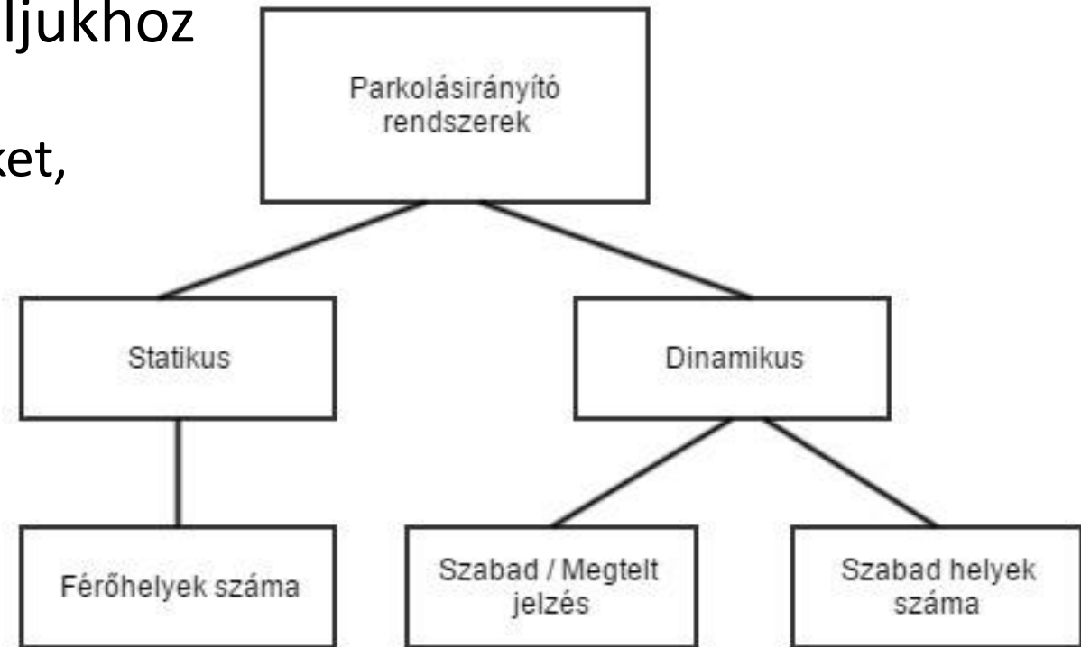
1. Ábra Parkolásirányító rendszerek felosztása (saját ábra)
